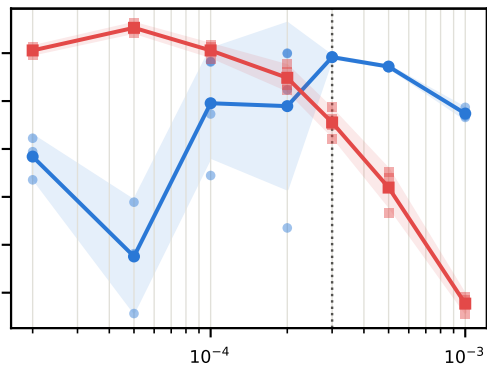
LoRA
