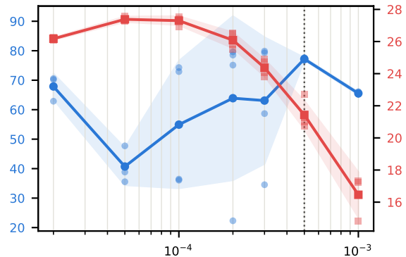
MiLoRA
