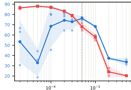
DoRA
